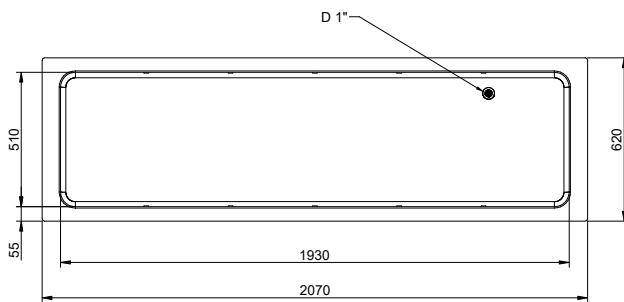
Boven aanzicht
